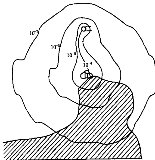
图 1 个体风险等值线示意图
