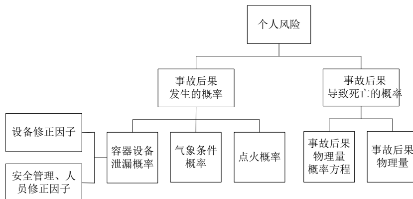
图 1 个体风险的计算程序
