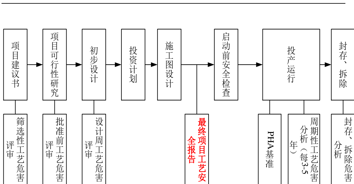
图 2 新疆华泰生产工艺风险辨识流程
