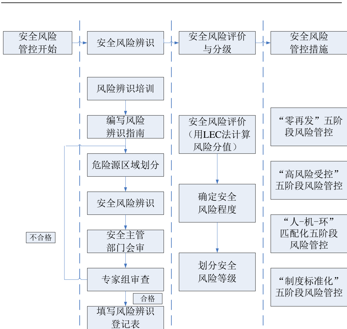
图 1 安全风险管控流程图
