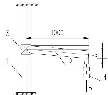
图 A.1.6-3 转动刚度试验示意图
