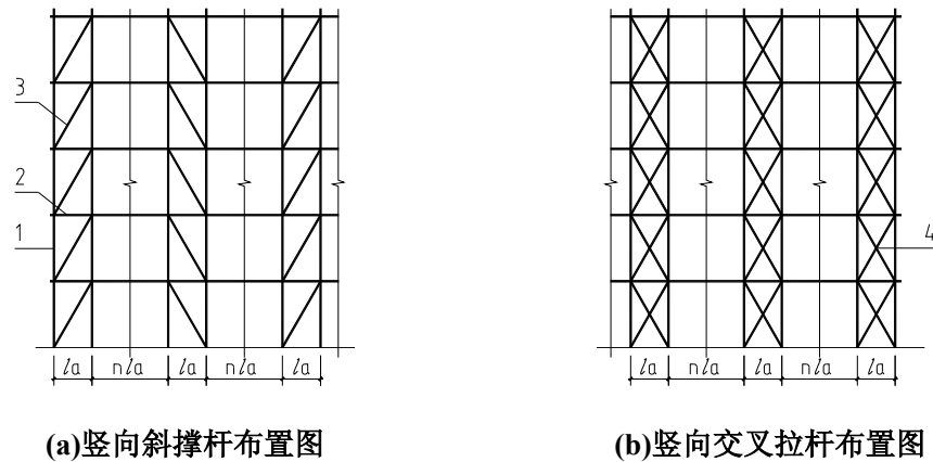
图 8.2.4 作业脚手架竖向斜撑杆布置示意图
